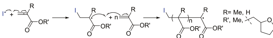
Esquema 3. Inicialización y propagación de la reacción de polimerización vía radicales libres de un monómero acrílico.
