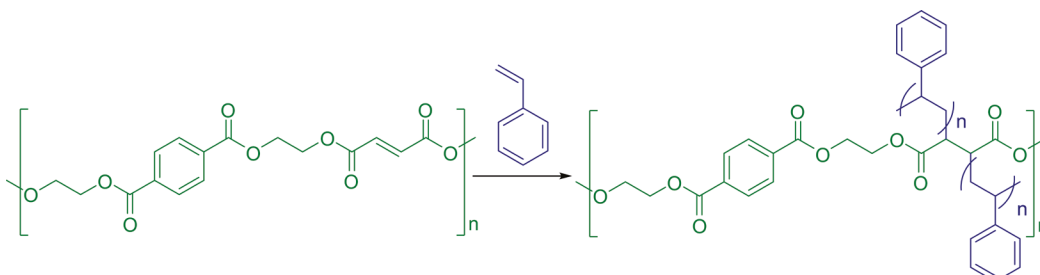
Esquema 6. Reacción de un poliéster insaturado con estireno.
