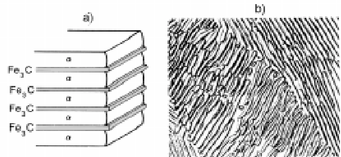
Figura 4. a) Esquema que permite ver el acoplamiento de las láminas de fase ferrita (α) con las de la fase cementita (Fe 3 C) para formar el microconstituyente perlitita; b) Perlitita amplificada 2,000 veces con microscopía óptica.
