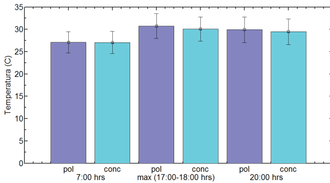
Figura 9. Promedio de temperaturas en el fondo de los depósitos de polietileno (pol) y concreto (conc) durante períodos de mañana (7 horas), noche (20 horas) y de máximas temperaturas (max (17:00-18:00 horas))
