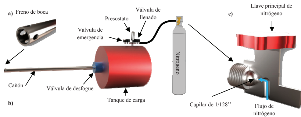
Figura 1. Diagrama del sistema de control de presión de gas, a) freno de boca, b) diagrama del sistema armado del cañón, c) capilar de control de flujo
