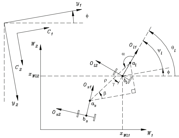
Figura 2. Vista de planta del sistema robótico
