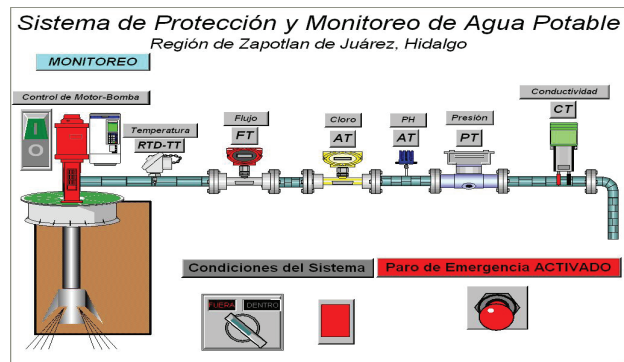
Figura 14. Sistema con HS_SISTEMA=0 y D_F_SISTEMA=0
