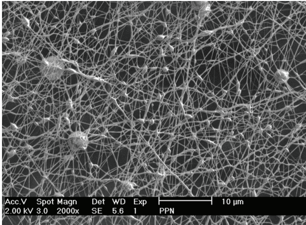
Figura 2. Imagen de MEB de fibras de polipirrol/óxido de polietileno/nylon-6 obtenidas por electrohilado a 2000x
