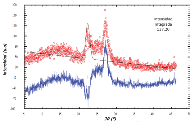
Figura 7. Intensidad integrada del pico 1 del patrón de difracción de polipirrol/óxido de polietileno/nylon-6
