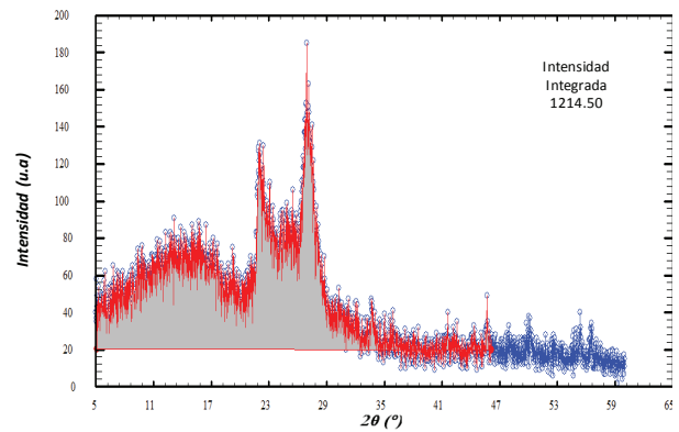
Figura 6. Intensidad integrada de la porción amorfa y porción cristalina de polipirrol/óxido de polietileno/nylon-6
