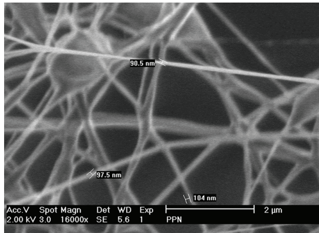
Figura 3. Imagen de MEB de fibras de polipirrol/óxido de polietileno/nylon-6 obtenidas por electrohilado a 16000x
