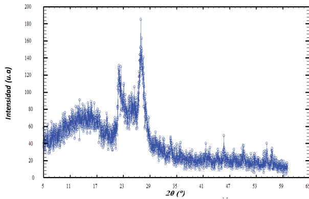
Figura 5. Patrón de difracción de microfibras de polipirrol/óxido de polietileno/nylon-6
