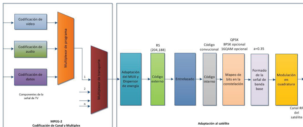
Figura 2. Estándar DVB-DSNG
