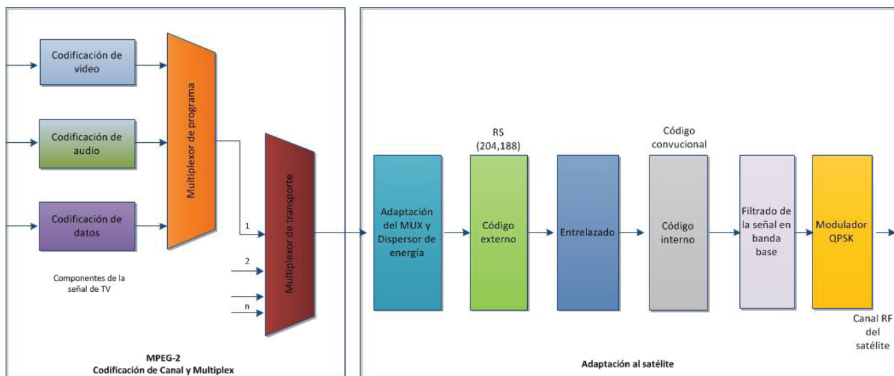
Figura1. Estándar DVB-S
