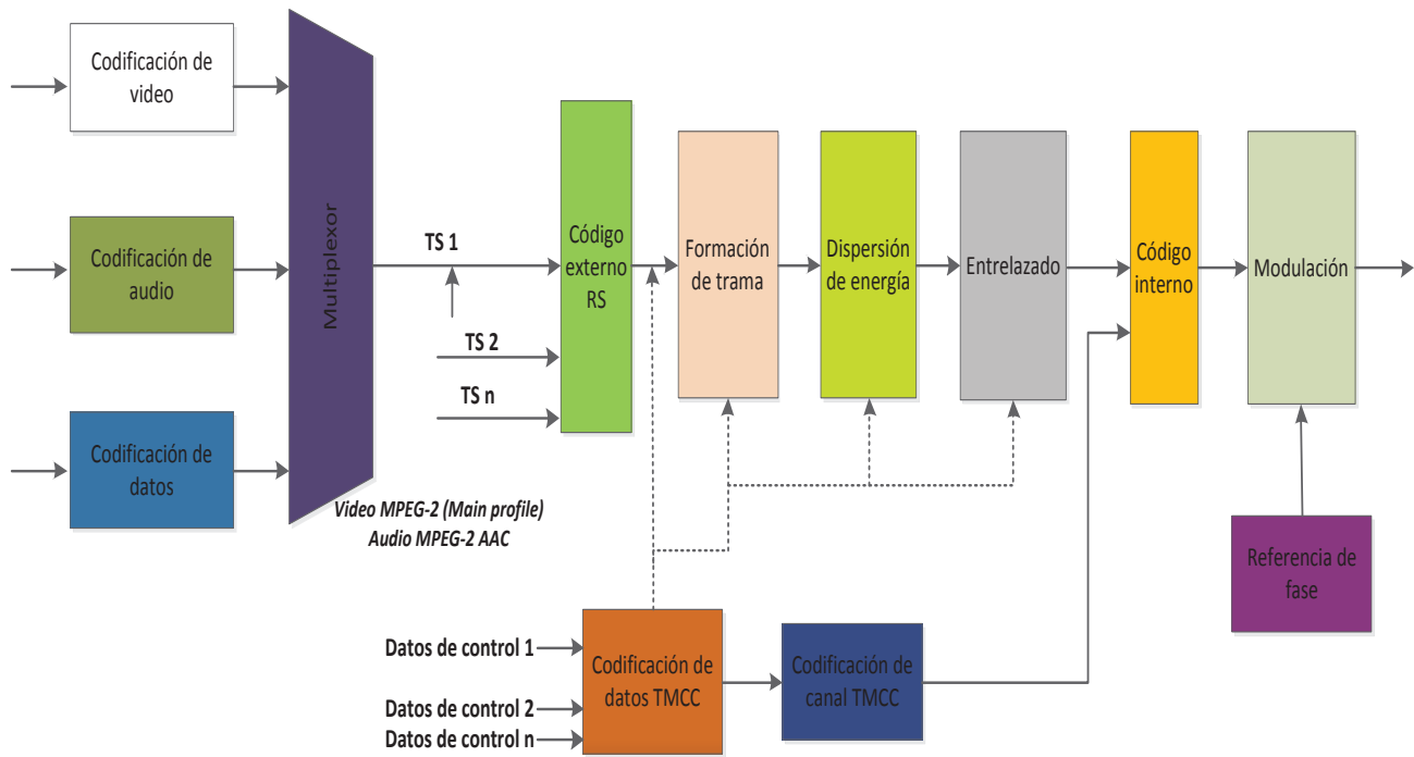
Figura 6. Estándar ISDB-S
