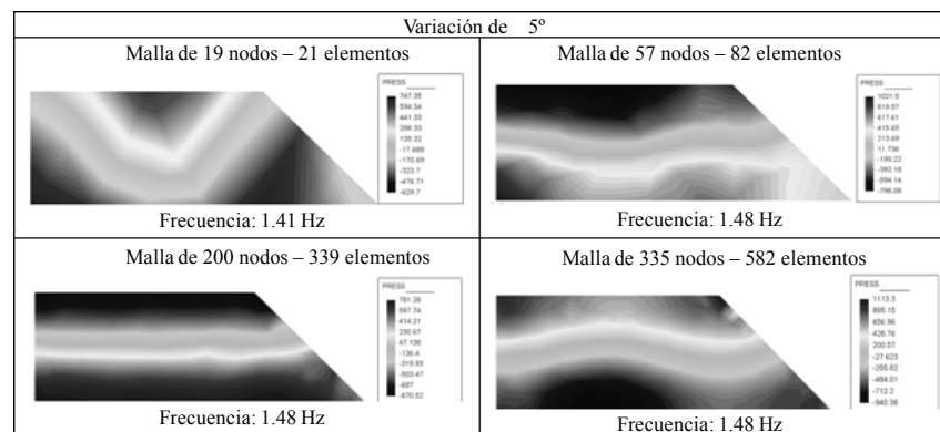
Figura 6. Cuarto modo de presión. Variación de \pm 5^\circ en la dirección normal al contorno
