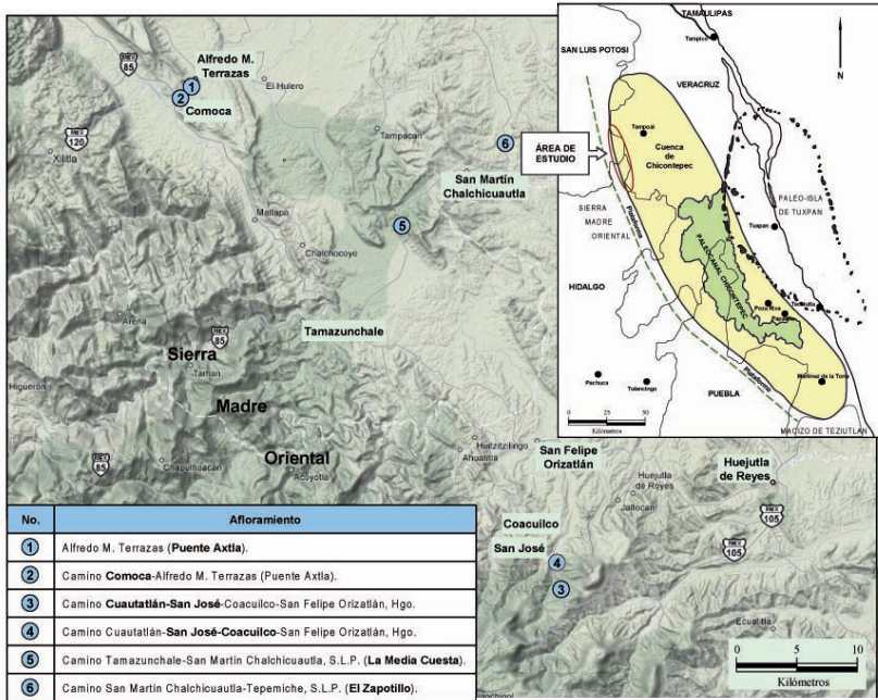
Figura 5. Localización de los afloramientos visitados dentro de la Cuenca de Chicontepec (Modificada y complementada de Google-Imágenes (2009) y Schlumberger (1984))
