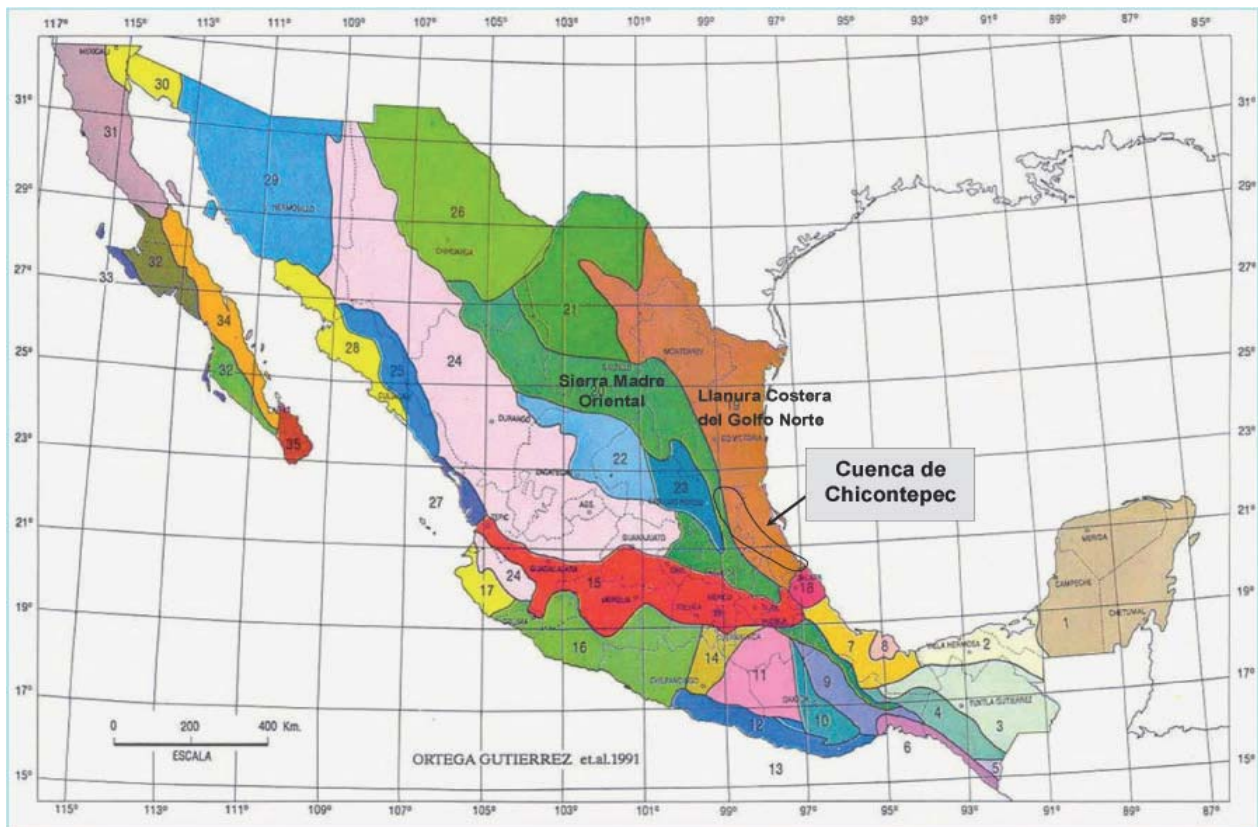
Figura 1. Provincias Geológicas de la Republica Mexicana: 1. Plataforma de Yucatán, 2. Cuenca Deltaica de Tabasco, 3. Cinturón chiapaneco de pliegues y fallas, 4. Batolito de Chiapas, 5. Macizo Ígneo del Soconusco, 6. Cuenca de Tehuantepec, 7. Cuenca Deltaica de Veracruz, 8. Macizo volcánico de los Tuxtlas, 9. Cuicateca, 10. Zapoteca, 11. Mixteca, 12. Chatina, 13. Juchateca, 14. Plataforma de Morelos, 15. Faja volcánica transmexicana, 16. Complejo Orogénico de Guerrero-Colima, 17. Batolito de Jalisco, 18. Macizo Ígneo de Palma Sola, 19. Migeoclinal del Golfo de México, 20. Cinturón mexicano de pliegues y fallas, 21. Plataforma de Coahuila, 22. Zacatecana, 23. Plataforma de Valles-San Luis Potosí, 24. Faja Ignimbrítica mexicana, 25. Cinturón Orogénico sinaloense, 26. Chihuahuense, 27. Cuenca de Nayarit, 28. Cuenca Deltaica de Sonora-Sinaloa, 29. Sonorense, 30. Delta del Colorado, 31. Batolito de Juárez-San Pedro Mártir, 32. Cuenca de Vizcaíno-Purísima, 33. Cinturón orogénico de Cedros-Margarita, 34. Faja volcánica de La Giganta, y 35. Complejo Plutónico de La Paz. Complementada de Ortega et al. (1992)
