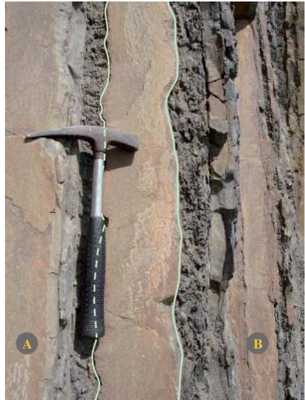
Foto 4.3. Estructura de carga de las areniscas sobre las arcillas por asentamientos diferenciales (vista de perfil) (A: base, B: cima) (martillo como escala: 31.8 cm)
