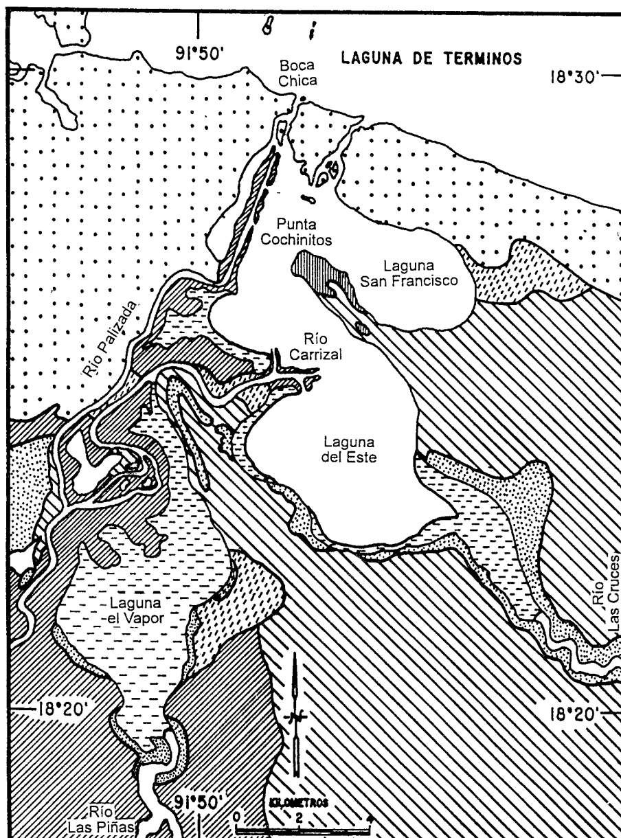
Fig. 2. Mapa de distribución generalizada de las comunidades vegetales del sistema fluvio-lagunar-deltaico del río Palizada. Tula(/////); carrizal (|||||); comunidad de Typha-Phragmites (.....); popal(xxxx); comunidad de Vallisneria americana (- - - -); manglar en el canal de Boca Chica (::); manglar de Punta Cochinitos (||||); manglar dominado por Rhizophora mangle (: : :).
