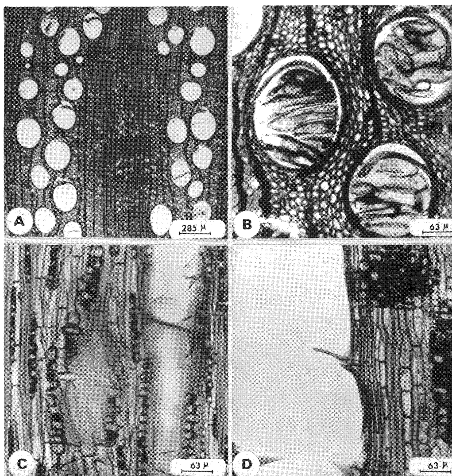
Fig. 2. Quercus laurina . A. Corte transversal 2.5 X. Porosidad difusa a semianular. B. Corte transversal 10 X. Vasos con túldes. C. Corte tangencial 10 X. Vasos con platina de perforación. D. Corte radial 10 X. Vaso y parénquima axial.
