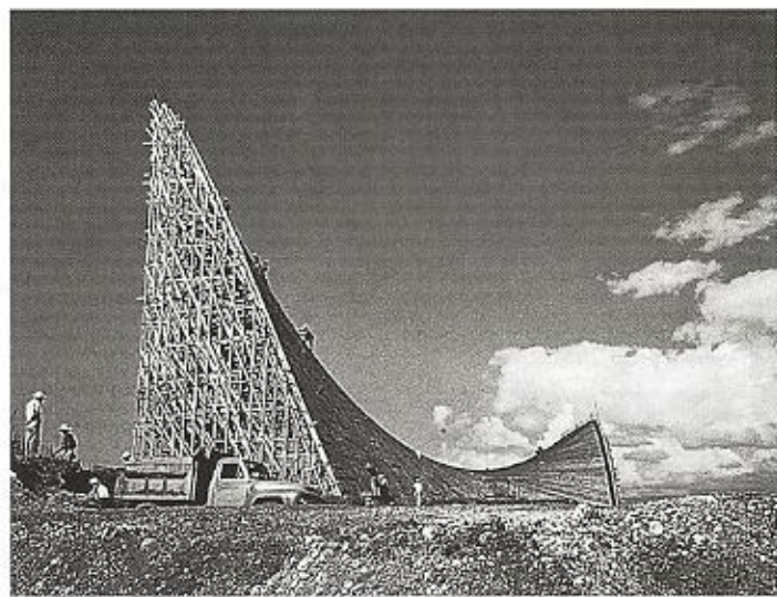
Cimbra en la ejecución original de la Capilla abierta de Palmira, Cuernavaca, Morelos, 1958-59. Arquitectos: Guillermo Rosell y Manuel Larrosa.
