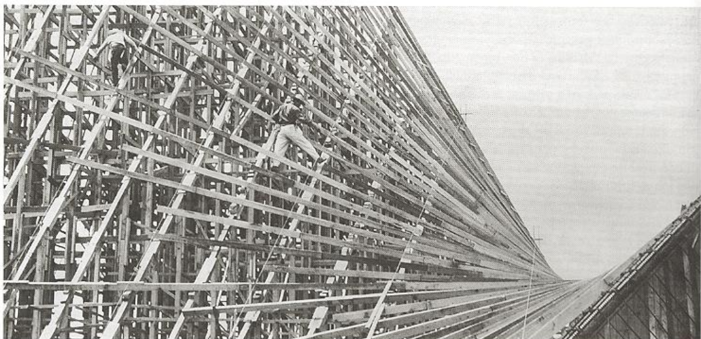
Cimbra para el cascarón de la capilla abierta de Palmira (1958).
