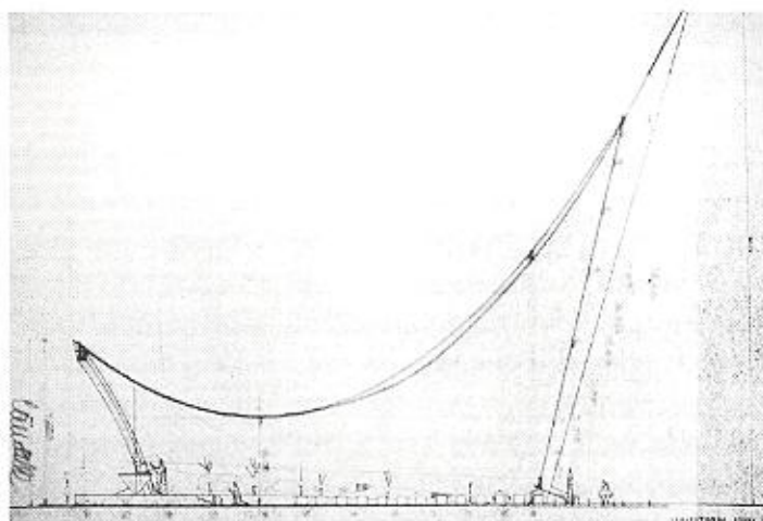
Proyecto reformado para la iglesia de Cuernavaca. Fechado en México D.F., febrero de 1958. Archivo Candela, Avery Library, Universidad de Columbia, Nueva York.
