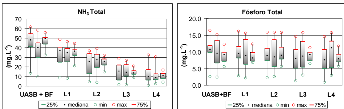
Figura 3 - Variações das concentrações de amônia e de fósforo total ao longo do sistema de tratamento nos três períodos operacionais.
