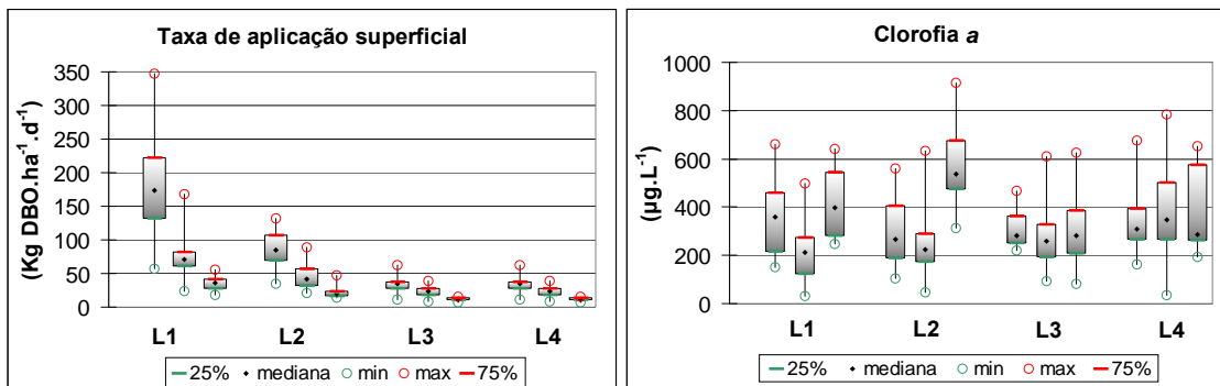
Figura 1 – Variações da taxa de aplicação superficial e das concentrações de clorofila a ao longo do sistema de tratamento nos três períodos operacionais.
