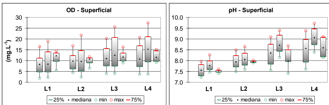
Figura 2 - Variações das concentrações de oxigênio dissolvido e do pH, medidos na superfície das lagoas, ao longo do sistema de tratamento nos três períodos operacionais.
