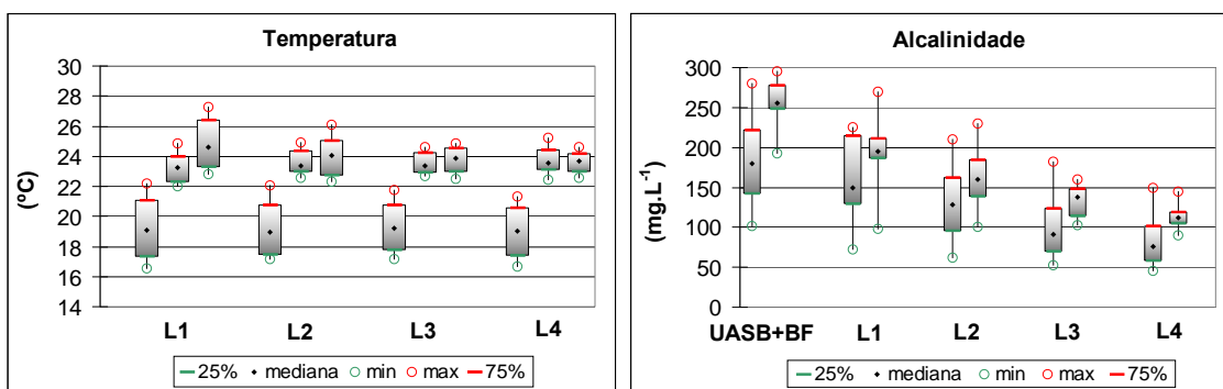
Figura 4 - Variações de temperatura nos três períodos operacionais e das concentrações de alcalinidade ao longo do sistema de tratamento nos Períodos 2 e 3 .
